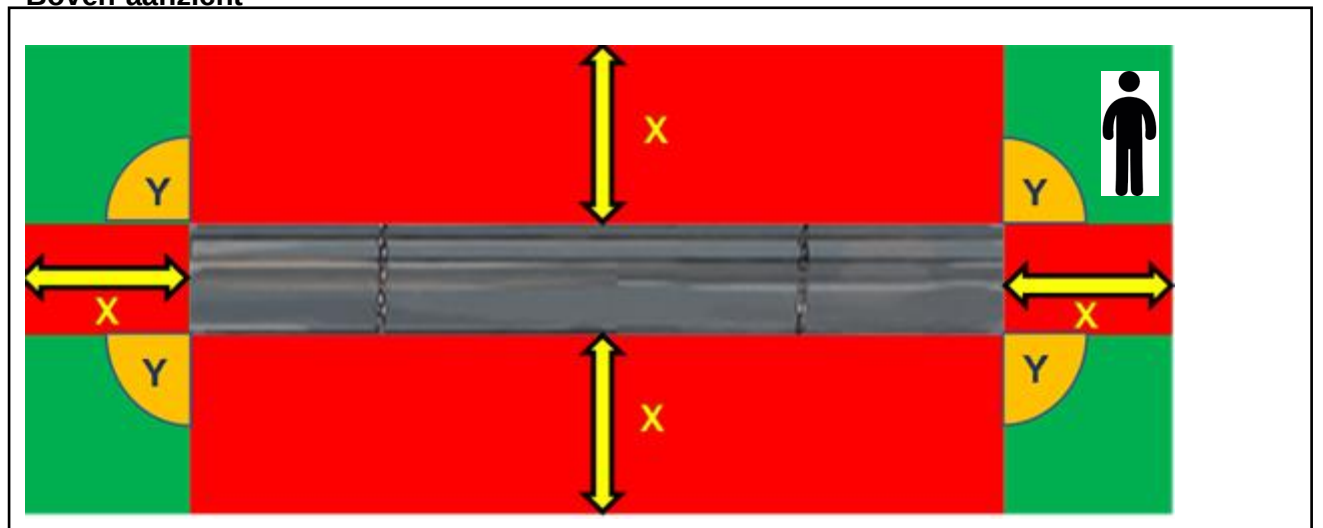
Boven-aanzicht
